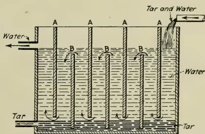
FIG. 73.—Baffle-Plate Tar Separator.
